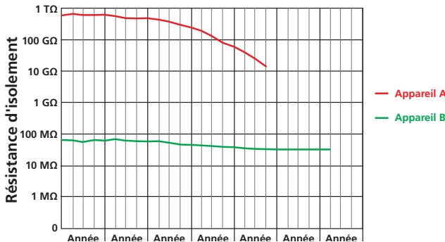
Fig 11 : Graphique du taux de résistance d'isolement
