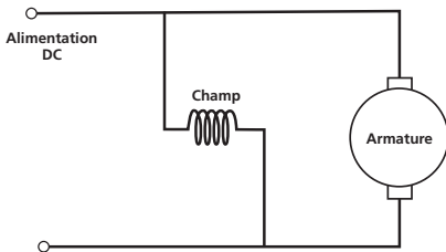
Fig 4 : Moteur DC à excitation parallèle
