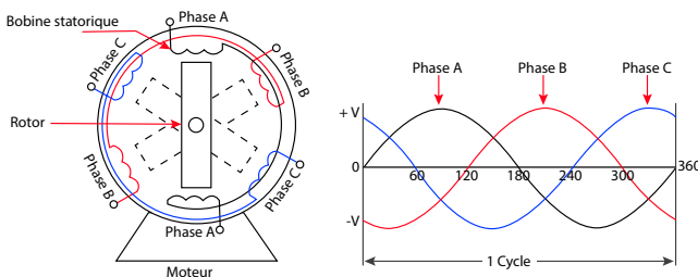
Fig 7 : Moteur triphasé
